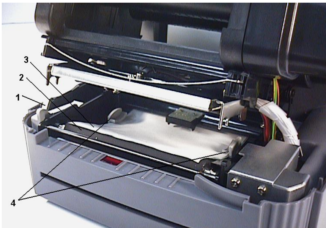
Figura 6. Alimentazione etichette mediante apposita guida regolabile
