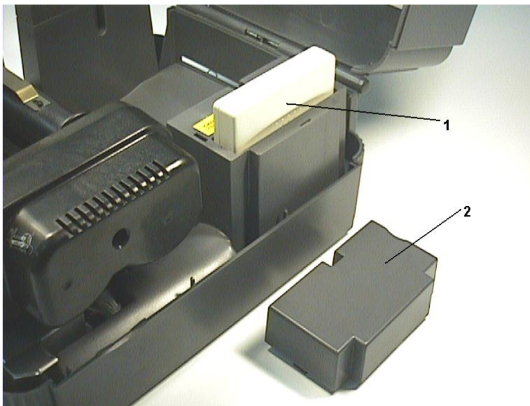
Figura 12. Installazione del modulo di memoria (opzionale)
